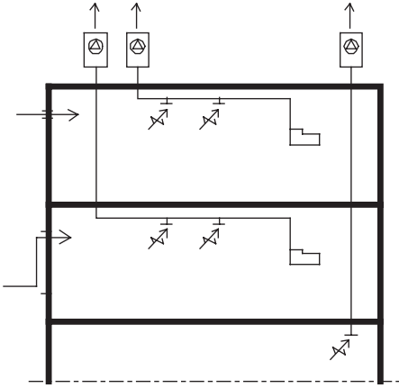
Kuva 1. Keskitetty, koneellinen tulo- ja poistoilmanvaihto, jossa on poistoilman lämmöntalteenotto tuloilmaan.
