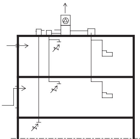
Kuva 4. Huoneistokohtainen, koneellinen poistoilmavaihto. Korvausilmalla voidaan ottaa talteen ikkunan lämpöhäviöt. Poistoilman lämmöntalteenottoon ei ole mielekkäitä kaupallisia tuotteita, mutta ilmanvaihtoa voidaan käyttää tarpeenmukaisesti.
