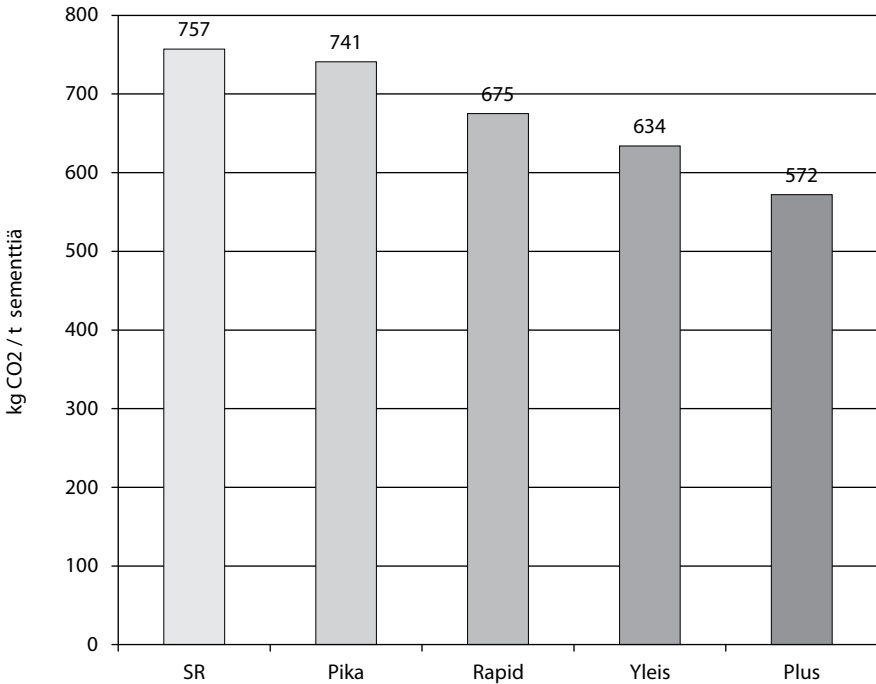
Kuva 3. Finnsementti Oy:n sementtien (Lappeenrannan tehdas) hiilidioksidipäästöt vuonna 2013 sementtitonnia kohti sementtilaaduittain esitettyinä.
