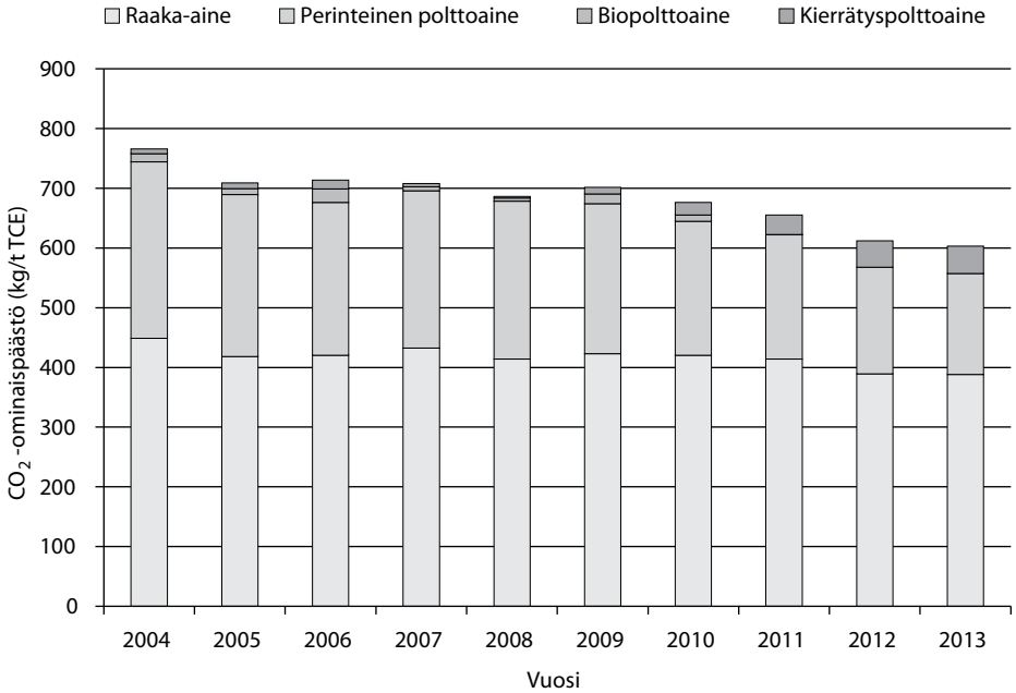
Kuva 1. Suomalaisen sementin valmistuksen hiilidioksidipäästöjen kehitys sementtitonnia kohti [4].
